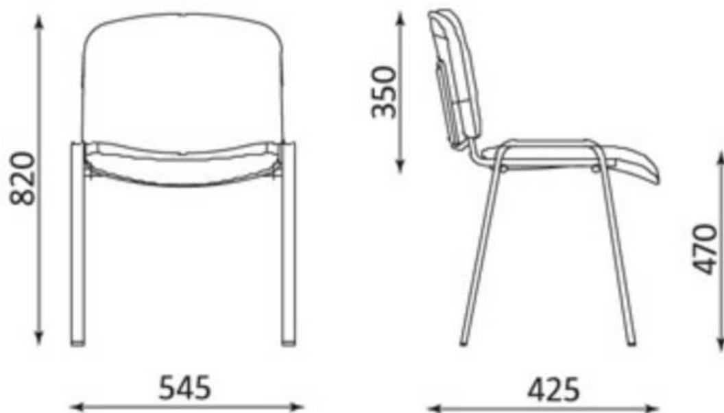
WYMIARY KRZESŁA KONFERENCYJNEGO ISO (kliknij na zdjęcie)
